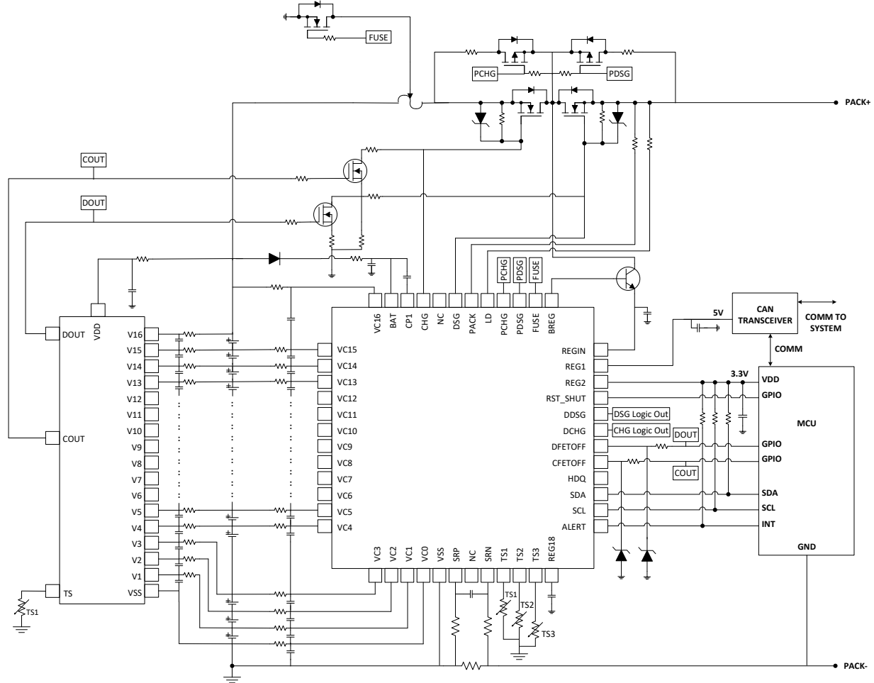
图 8-4. BQ77207 + BQ76952
