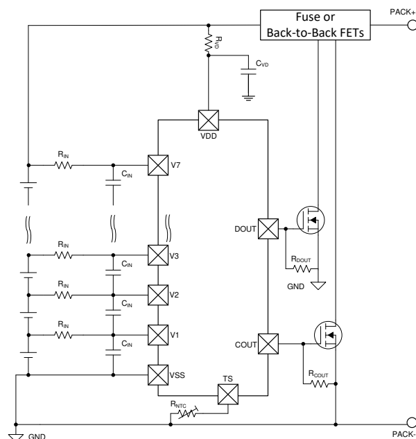
概略回路図
