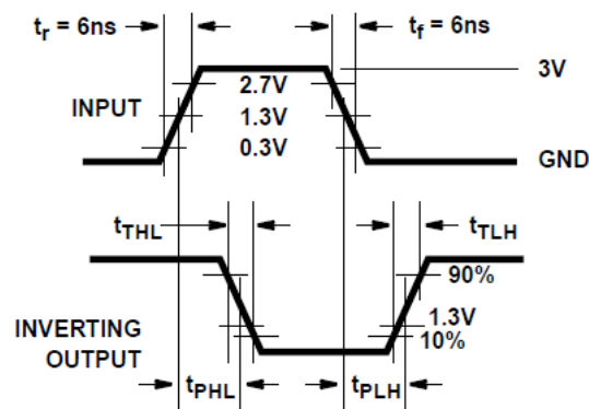
图 6-2. HCT 转换时间和传播延迟时间, 组合逻辑
