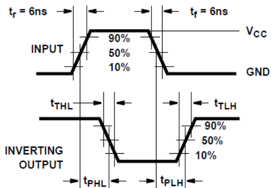
图 6-1. HC 和 HCU 转换时间和传播延迟时间, 组合逻辑
