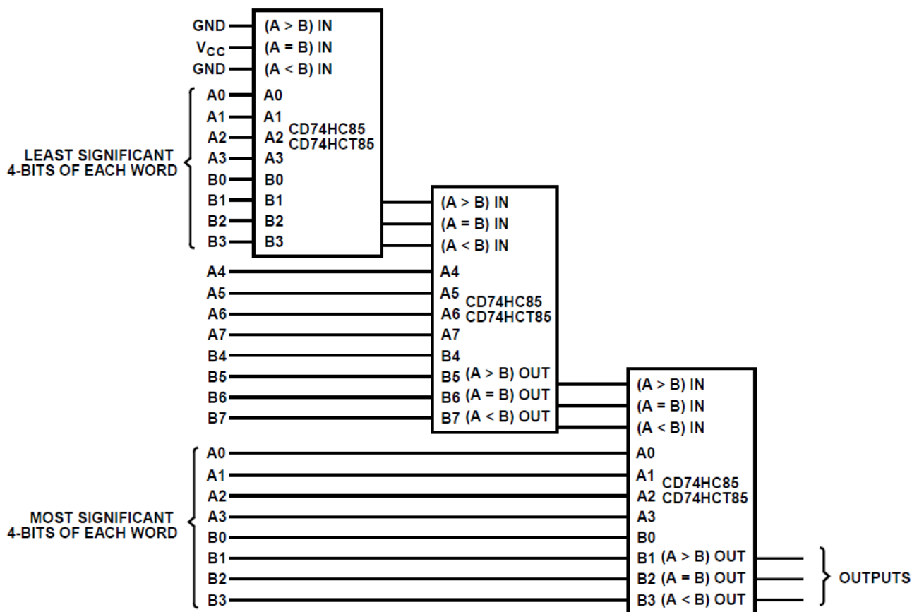
图 6-3. 级联 - 比较 12 位字
