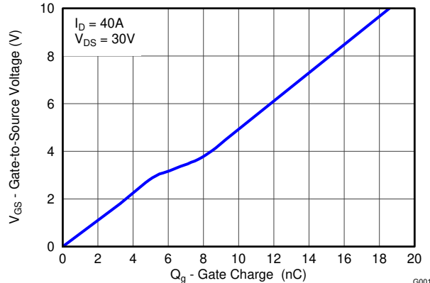
ゲート電荷
