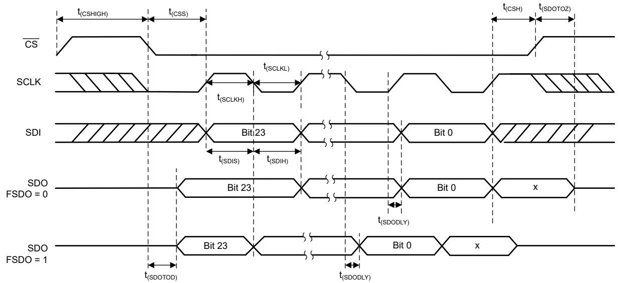
図 5-2. SPI Timing Diagram
