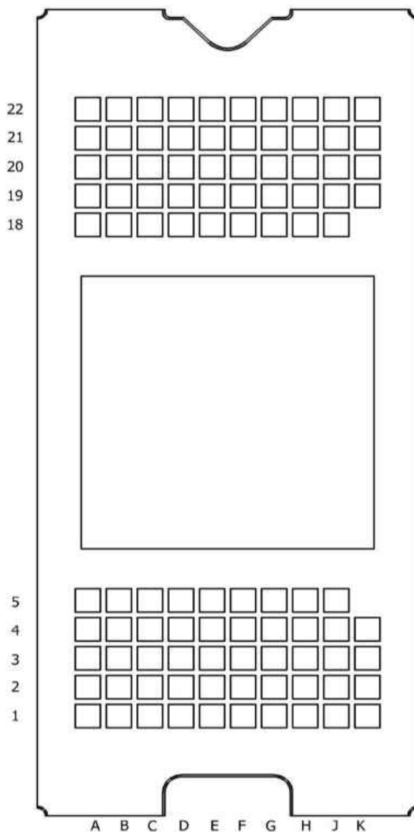
図 6-2. FQD Package LCCC (98) Bottom View
