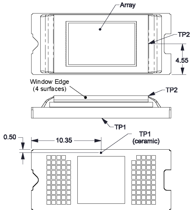
図 8-4. Thermal Test Point Location - FQD Package
