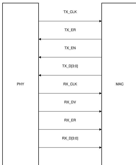
図 7-14. MII Signaling
