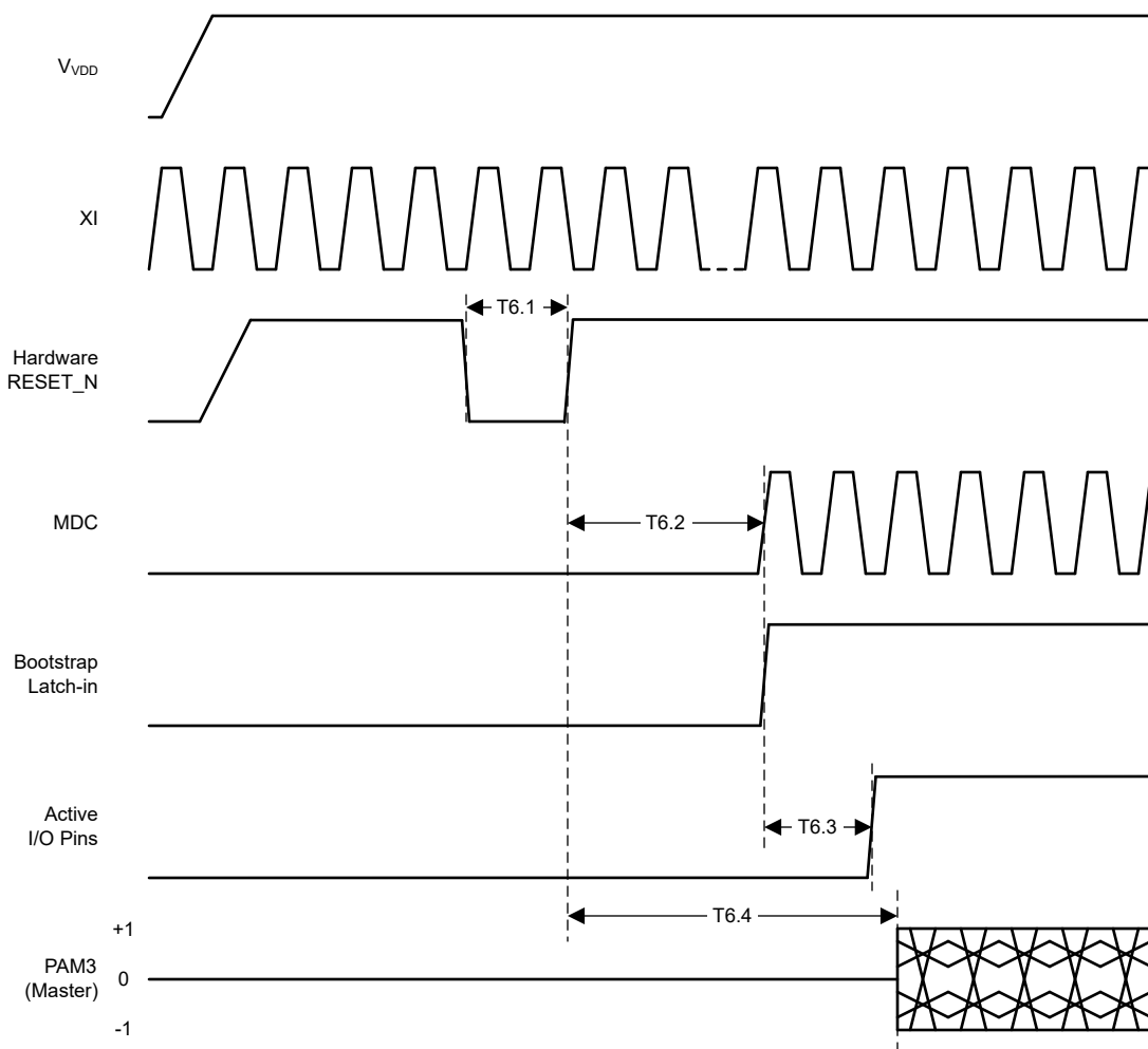
図 6-8. Reset Timing
