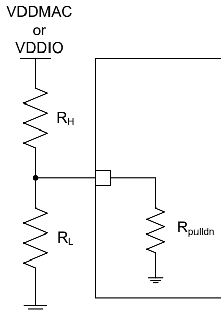
図 7-18. Strap Circuit
