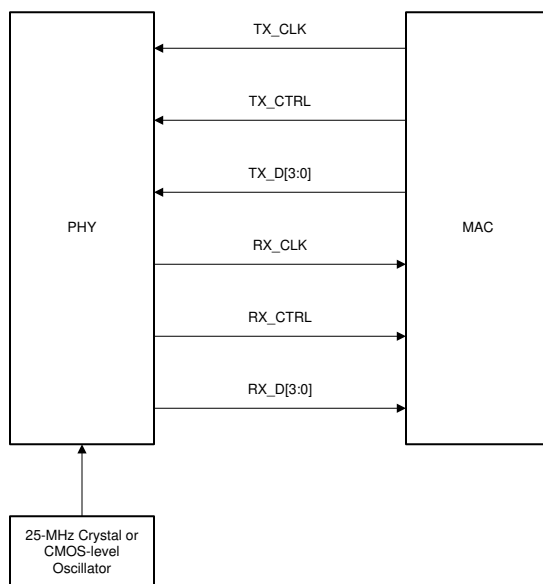
図 7-13. RGMII の接続
