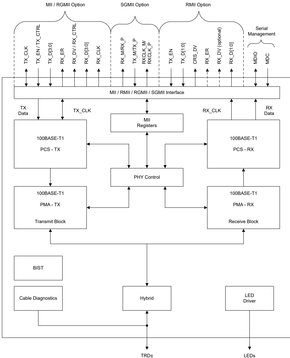
図 7-1. DP83TC814S-Q1
