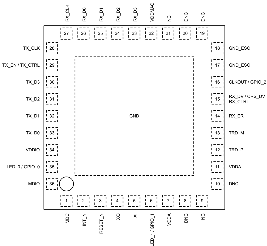
図 5-2. DP83TC814R-Q1 RHA パッケージ 36 ピン VQFN 上面図
