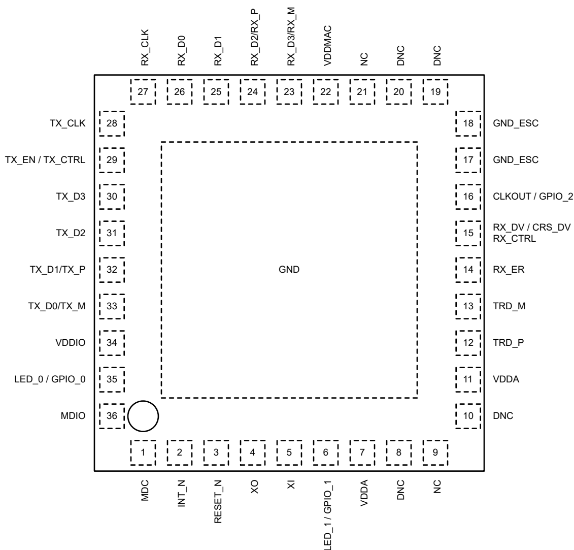
図 5-1. DP83TC814S-Q1 RHA パッケージ 36 ピン VQFN
