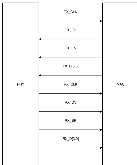
図 7-11. MII シグナリング
