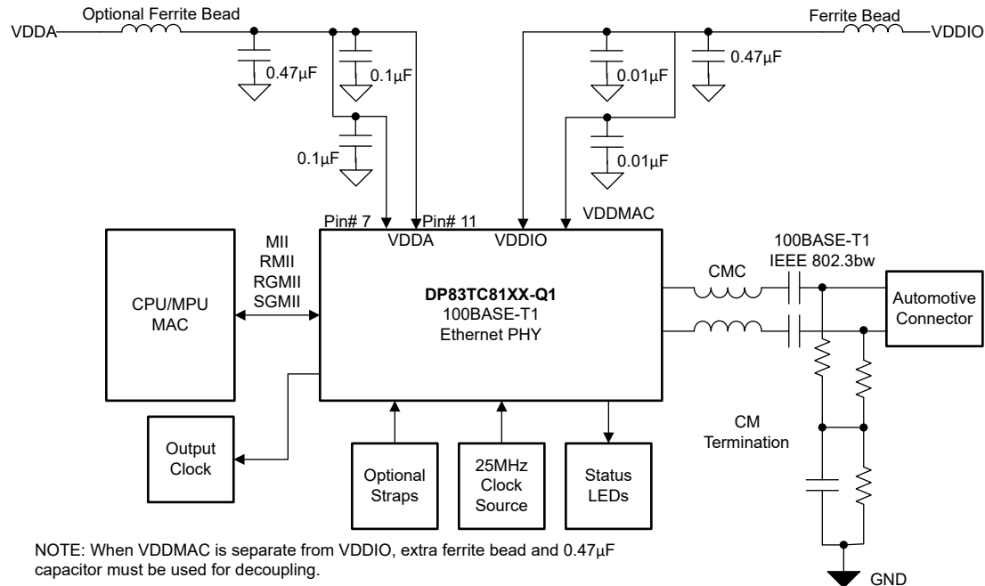
図 9-9. ペリフェラルを使用した代表的なアプリケーション
