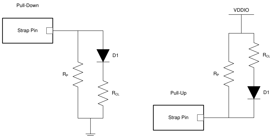
図 7-16. ストラップ接続の例
