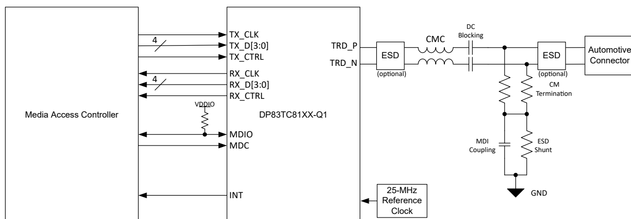
図 9-5. 代表的なアプリケーション (RGMII)
