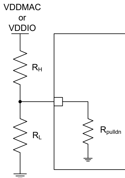
図 7-15. ストラップ回路
