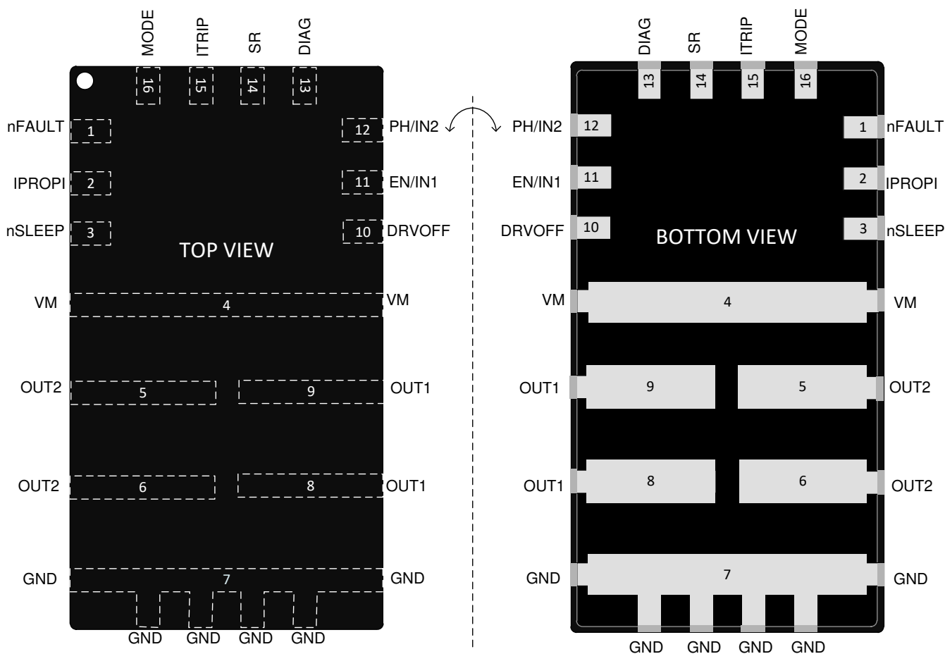
図 6-2. DRV8244H-Q1 HW バリエント、VQFN-HR (16) パッケージ
