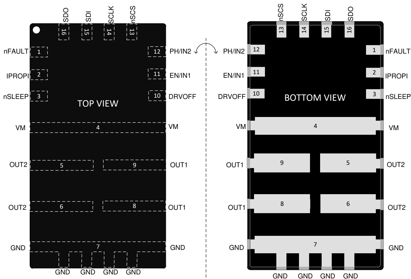
図 6-4. DRV8244S-Q1 SPI バリエント、VQFN-HR (16) パッケージ
