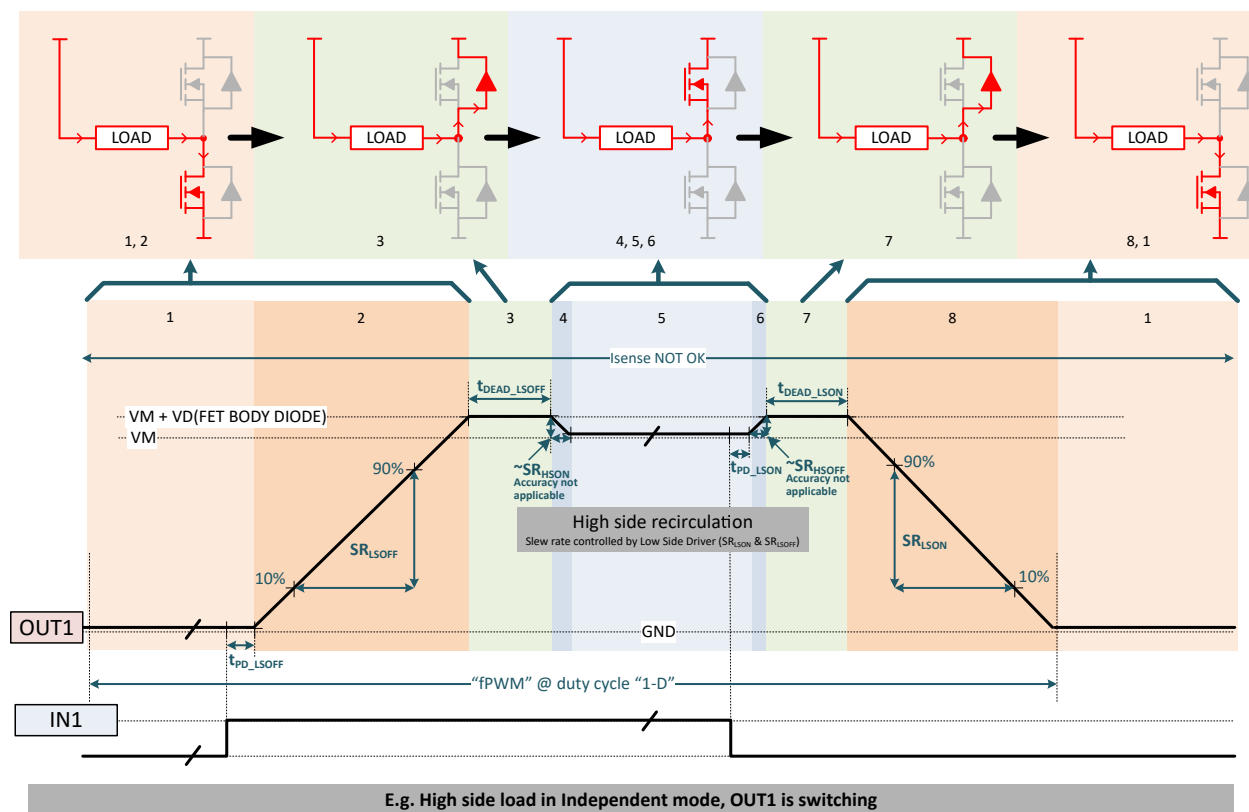
図 7-3. ハイサイド電流によるハーフブリッジの出力スイッチング遷移
