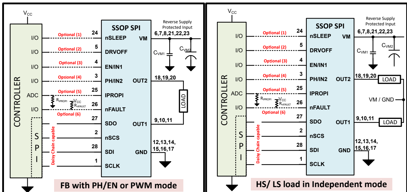
図 9-6. 代表的なアプリケーション回路図 - HVSSOP パッケージの SPI (S) バリエント
