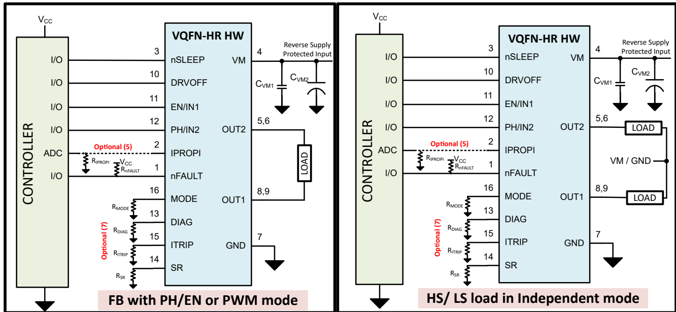
図 9-5. 代表的なアプリケーション回路図 - VQFN-HR パッケージの HW バリエント
