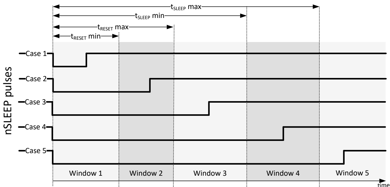
図 8-9. nSLEEP パルスのシナリオ
