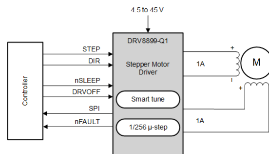
概略回路図
