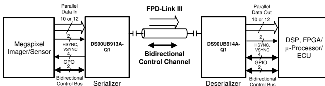
簡略回路図
