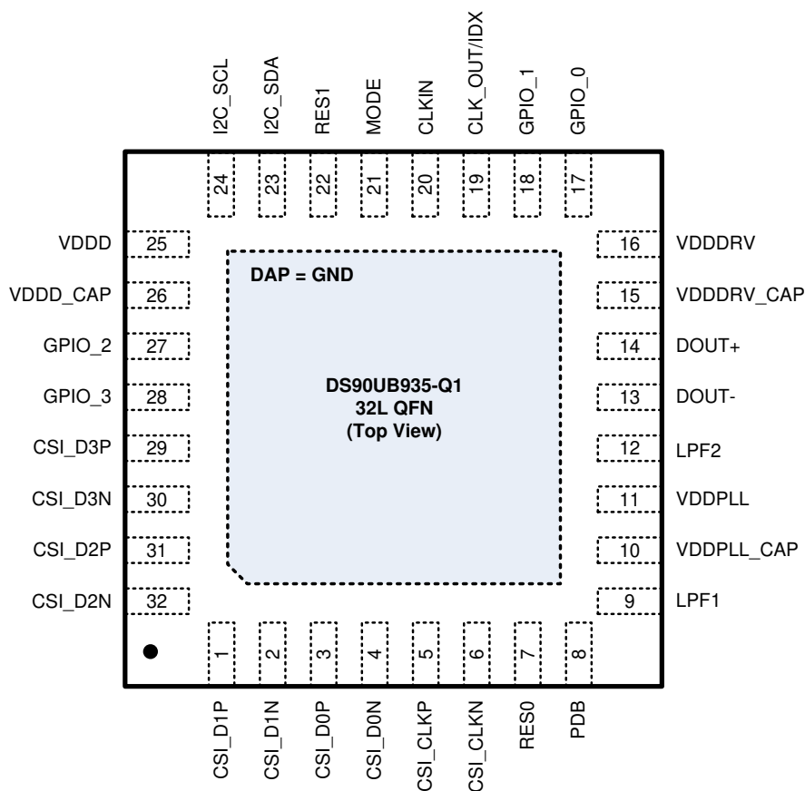
図 4-1. RHB パッケージ 32 ピン VQFN 上面図
