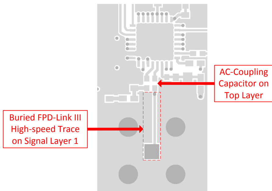
図 7-11. DS90UB935-Q1 シリアルライザ DOUT+ トレースのレイアウト
