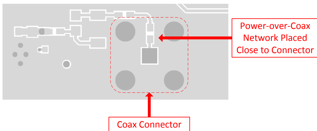
図 7-12. DS90UB935-Q1 同軸ケーブルを使用した電力供給 (Power-over-Coax) のレイアウト
