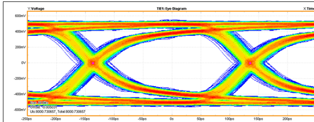
図 8. DOUT0 Eye at 3.675 Gbps
