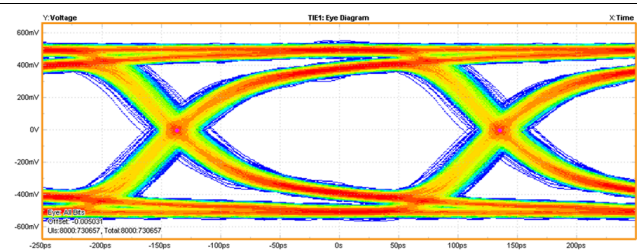
図 9. DOUT1 Eye at 3.675 Gbps
