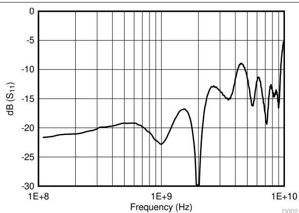
6-2. Return Loss
