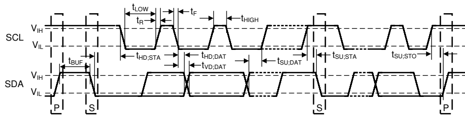
图 7-1. HDC302x I 2 C Timing Diagram
