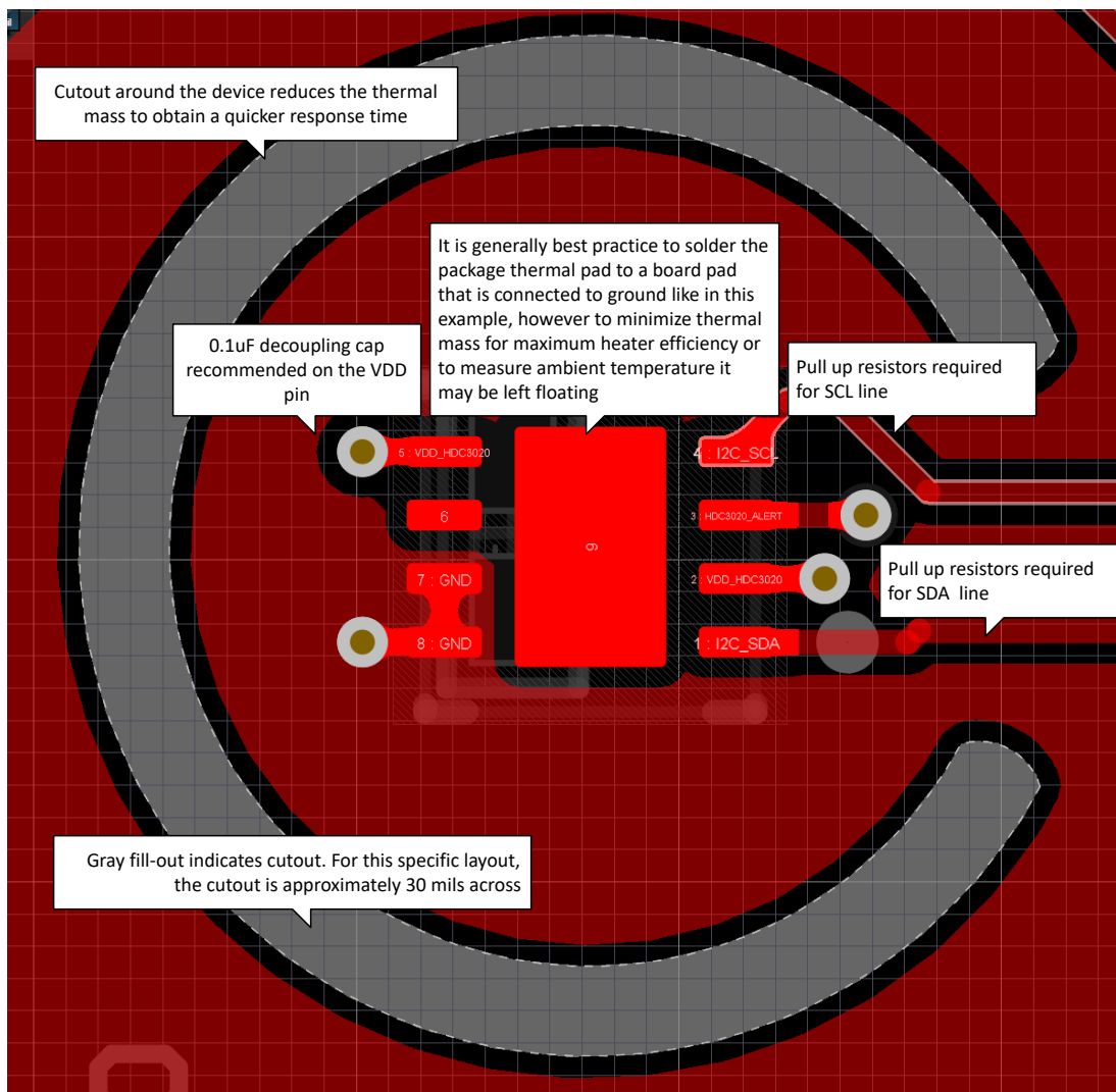
9-3. HDC302x PCB Layout Example
