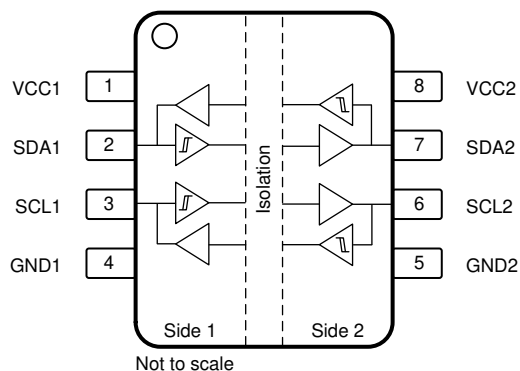
図 5-1. ISO1540-Q1 D Package 8-Pin SOIC Top View
