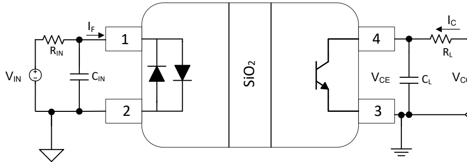
図 7-5. ISOM811[5-8]-Q1 帯域幅のテスト回路
