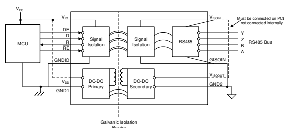
概略回路図
