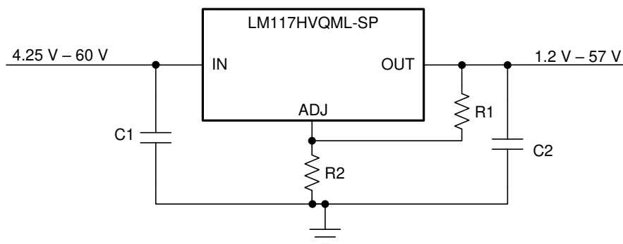
概略回路図
