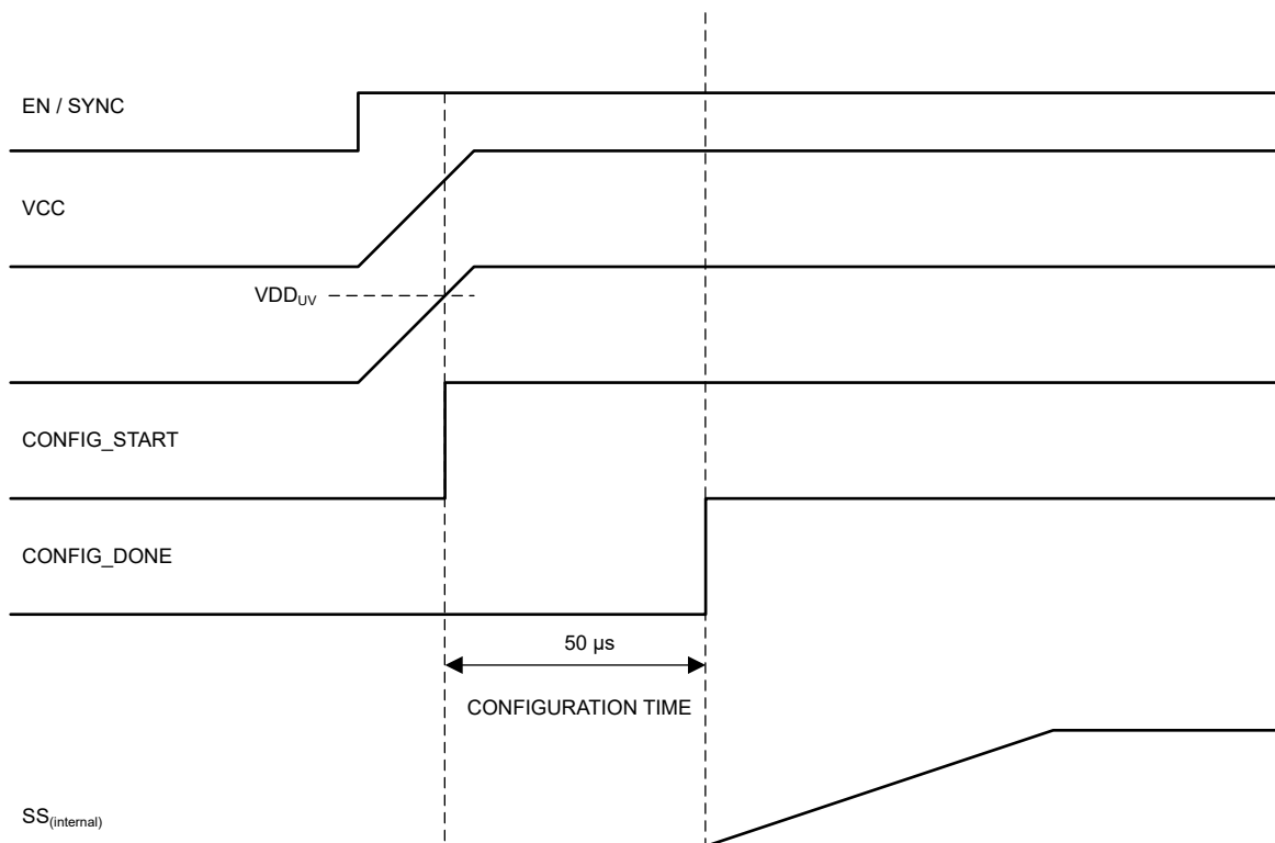
図 8-6. Configuration Timing
