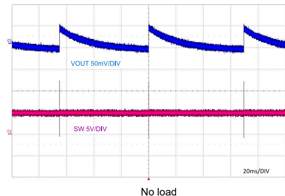
図 9-8. PFM Switching
