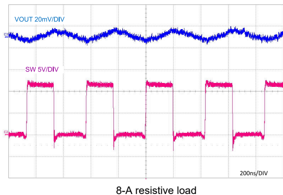
図 9-7. Full Load Switching
