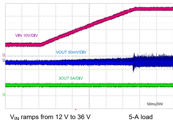
図 9-9. Line Transient
