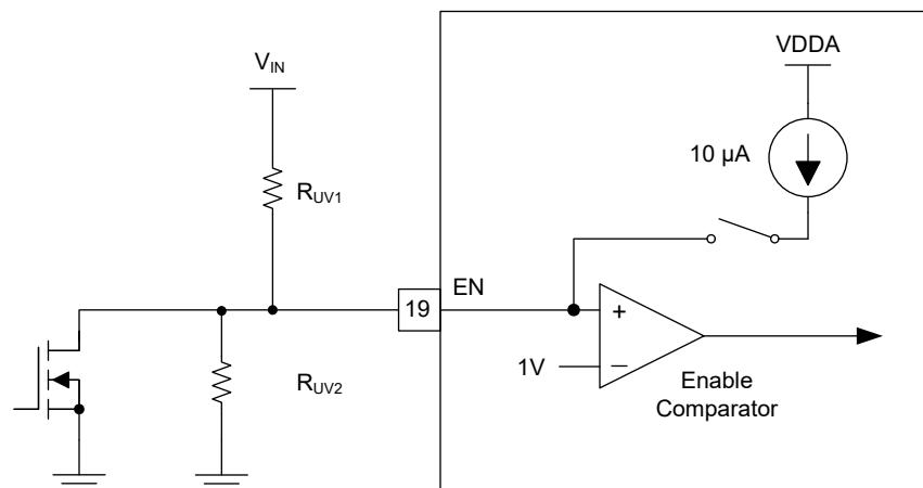
図 8-2. Programmable Input Voltage UVLO Turn-On
