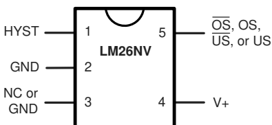
図 4-1. 5 リード SOT-23、DBV パッケージを参照
