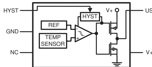
図 6-3. LM26CIM5 - __F
