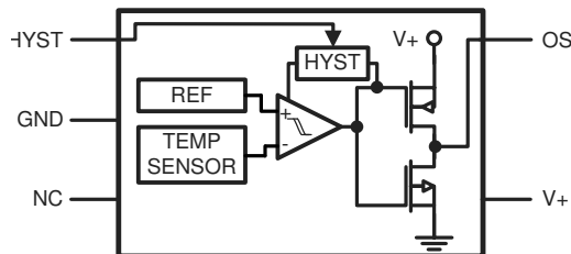
図 6-2. LM26CIM5 - __E
