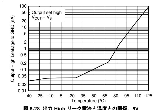
図 6-28. 出力 High リーク電流と温度との関係、5V
