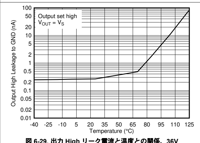
図 6-29. 出力 High リーク電流と温度との関係、36V
