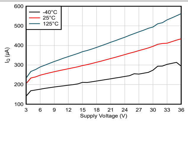
図 5-18. 静止電流と電源電圧との関係
