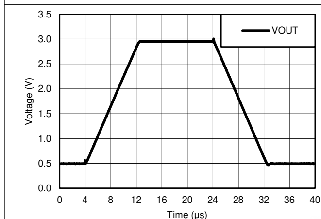
図 6-43. 電圧フォロワの大信号応答 (50pF)
