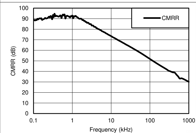
図 6-42. 同相除去比と周波数との関係
