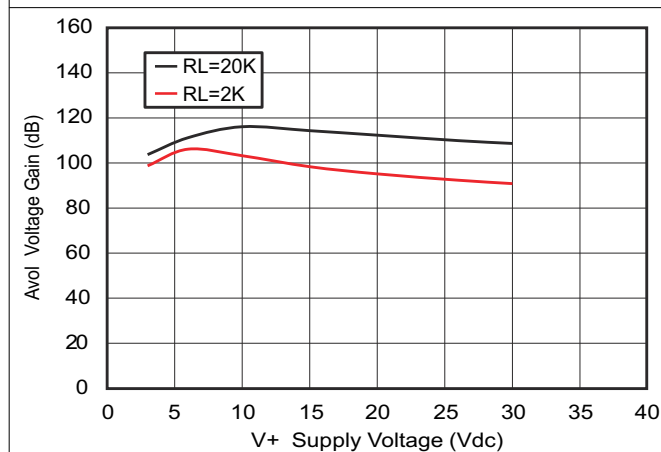
図 6-41. 電圧ゲインと電源電圧との関係
