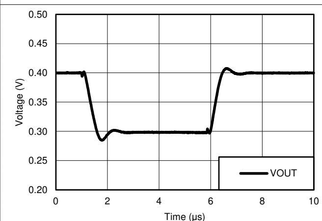
図 6-44. 電圧フォロワの小信号応答 (50pF)
