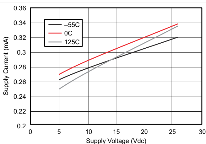
図 6-40. 消費電流と電源電圧との関係
