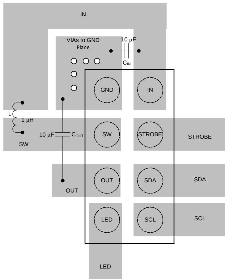
图 81. LM36010 Layout Example
