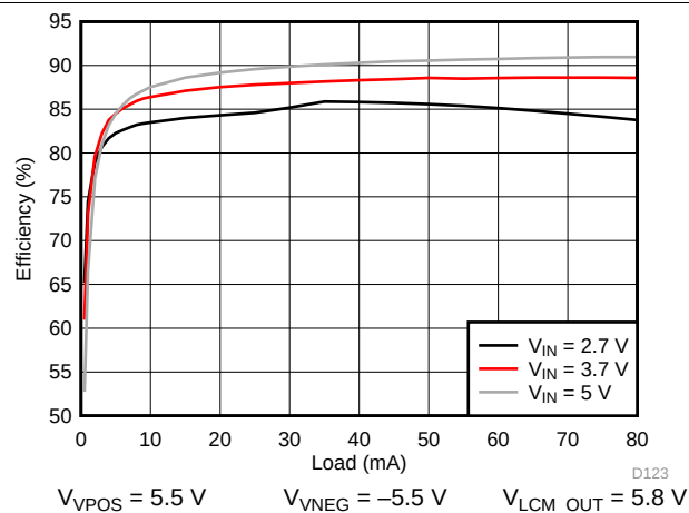
图 137. VPOS/VNEG Efficiency
