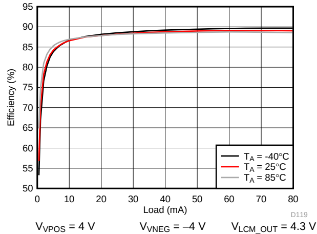
图 133. VPOS/VNEG Efficiency
