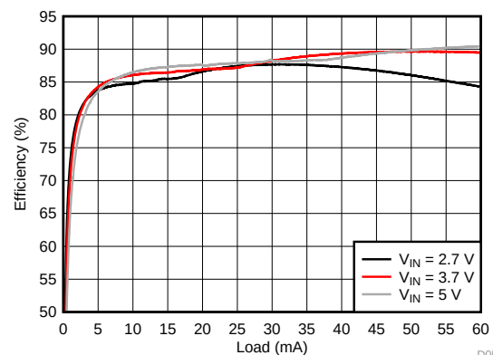
バックライト効率、2P8S
