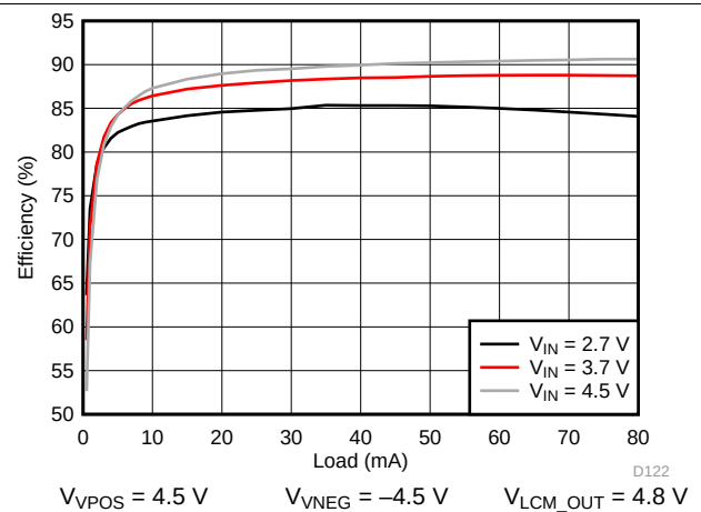
图 136. VPOS/VNEG Efficiency
