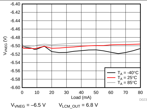
图 26. V_{NEG} Load Regulation
