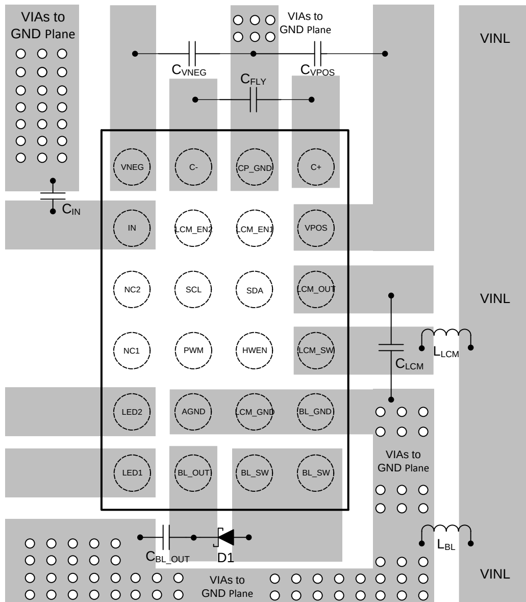
✎ 139. LM36272 Layout Example
