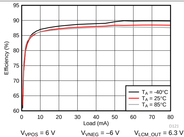
图 135. VPOS/VNEG Efficiency
