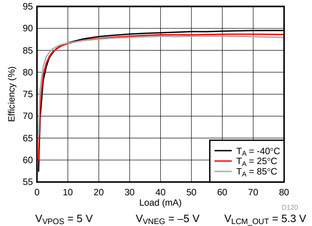
图 134. VPOS/VNEG Efficiency
