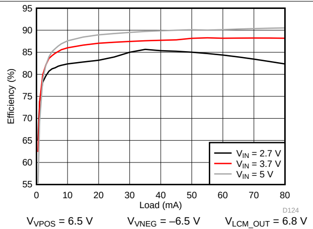
图 138. VPOS/VNEG Efficiency
