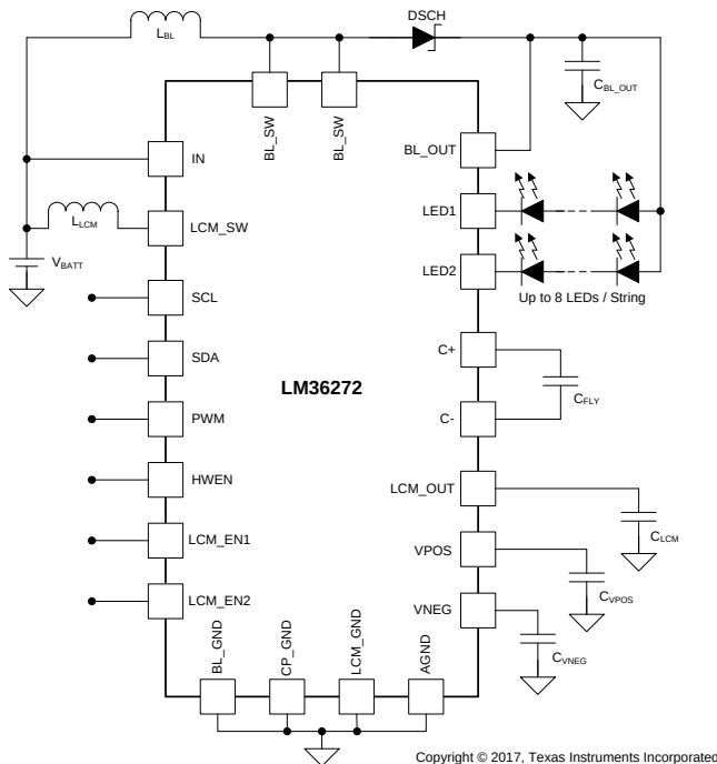
概略回路図
