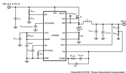
概略回路図
