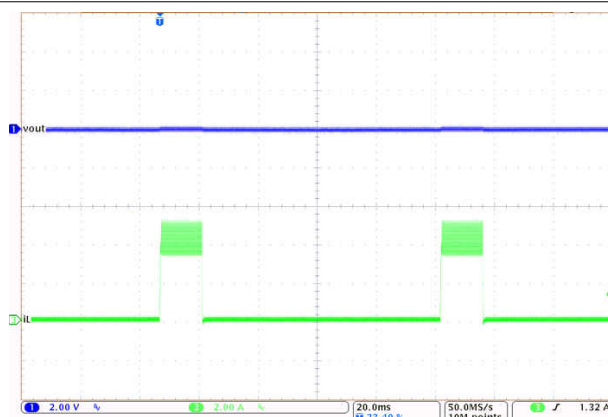
图 9-34. LM61430-Q1 Short Circuit Protection
