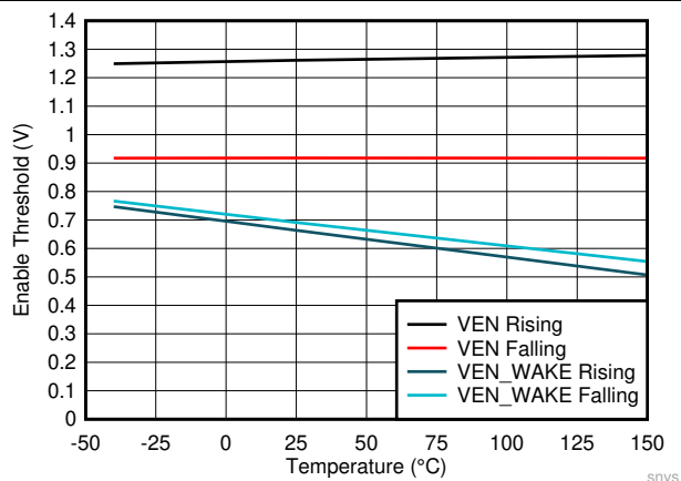
7-6. Enable Thresholds
