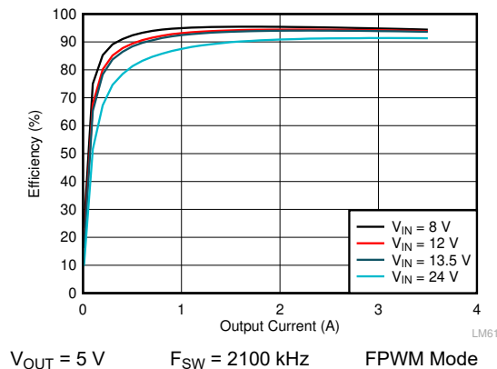
图 9-8. LM61435-Q1 Efficiency
