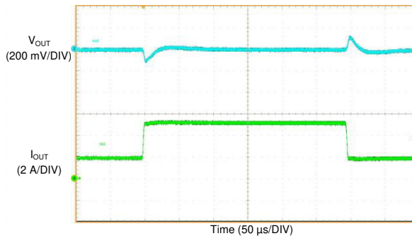
FIG 10-38. LM61460-Q1 Load Transient
