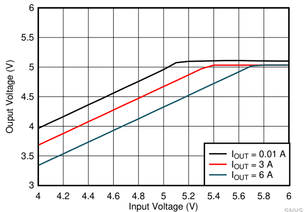
图 10-24. LM61460-Q1 Dropout Curve
