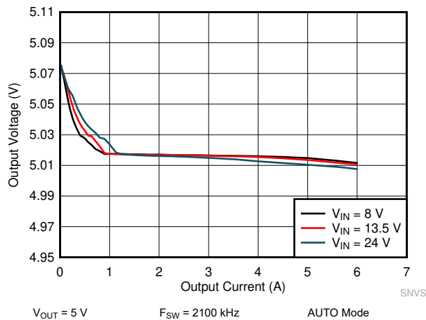
图 10-19. LM61460-Q1 Load and Line Regulation
