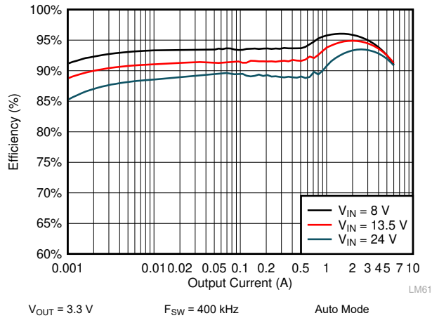
图 10-5. LM61460-Q1 Efficiency
