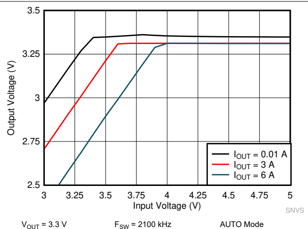
图 10-22. LM61460-Q1 Dropout Curve
