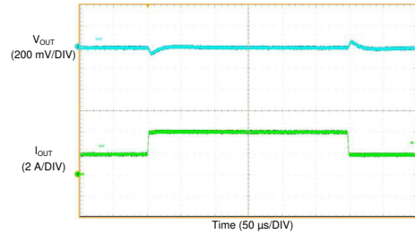
FIG 10-41. LM61460-Q1 Load Transient
