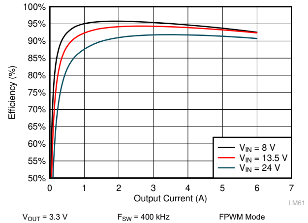
图 10-6. LM61460-Q1 Efficiency
