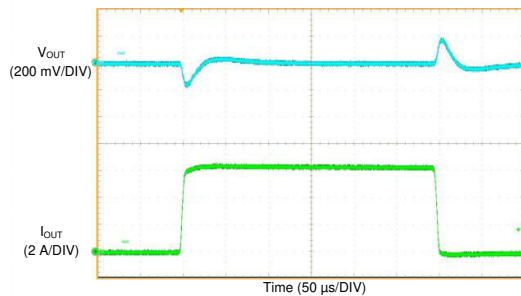
FIG 10-43. LM61460-Q1 Load Transient
