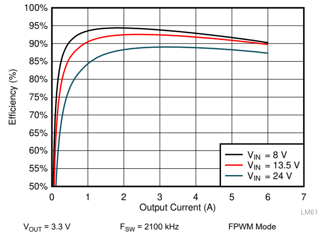
图 10-8. LM61460-Q1 Efficiency
