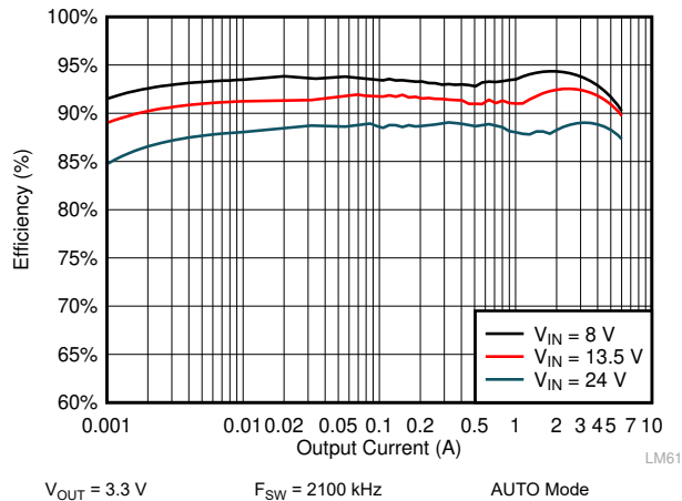
图 10-7. LM61460-Q1 Efficiency
