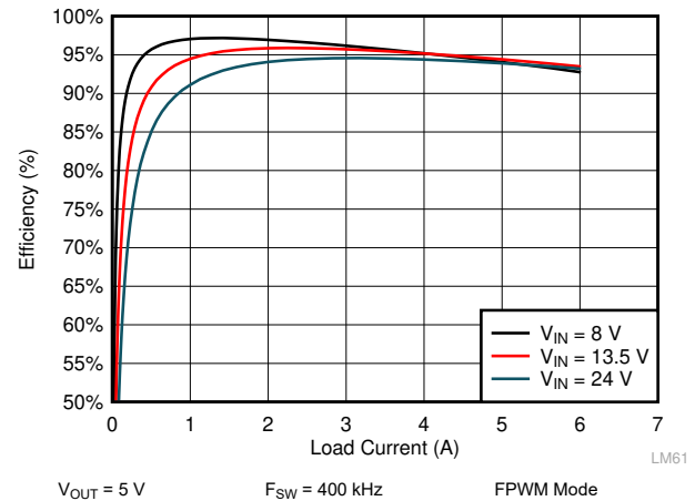
图 10-10. LM61460-Q1 Efficiency
