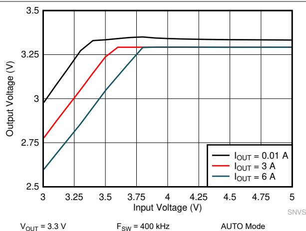
图 10-21. LM61460-Q1 Dropout Curve
