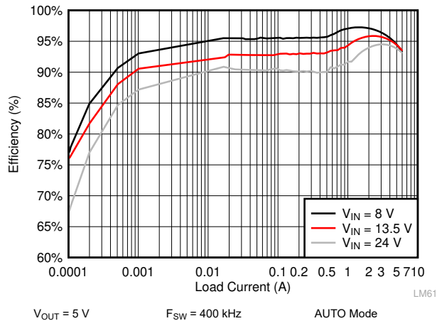
图 10-9. LM61460-Q1 Efficiency
