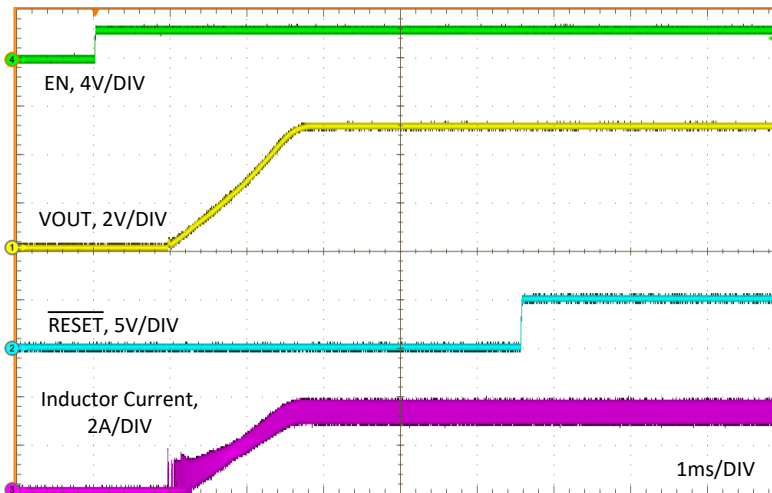
図 7-1. Precision Enable Behavior
