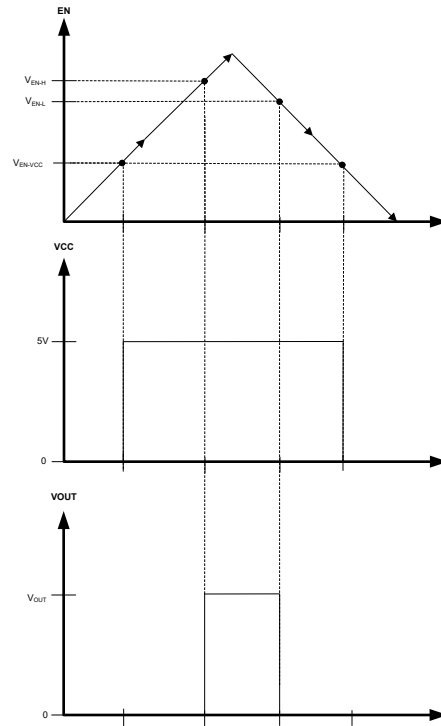
図 7-1. Precision Enable Behavior
