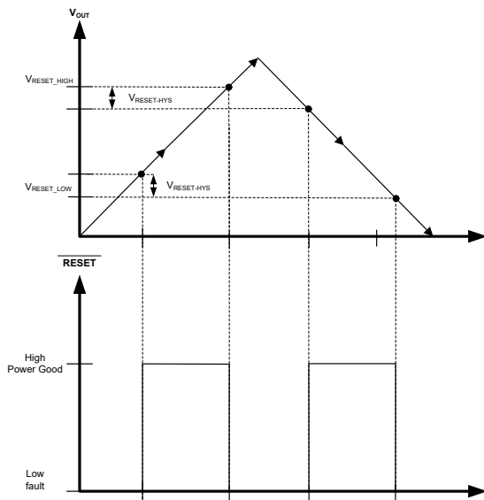
図 7-3. Static RESET Operation
