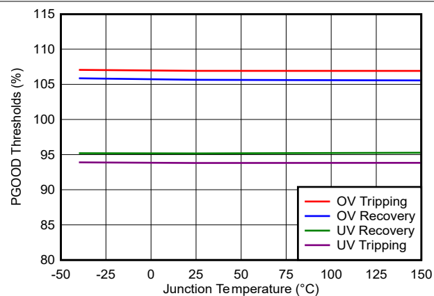
図 6-8. PGOOD スレッシュヨルド
