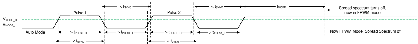
図 7-9. 自動モードから FPWM モードへの遷移でのスペクトラム拡散の無効化
