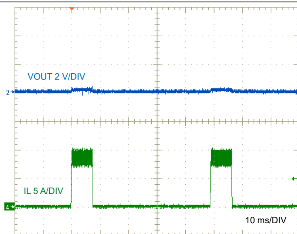
図 8-9. LM644x0-Q1 の短絡ヒック
