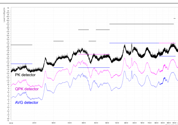
図 8-20. CISPR 25 Class 5 放射 EMI、 ログ アンテナ、垂直偏波、 200MHz ~ 1GHz
