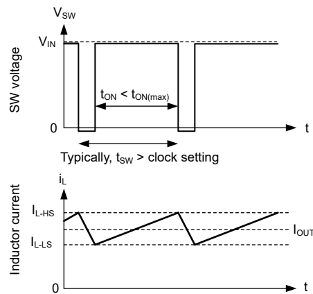
図 7-17. 電流制限波形
