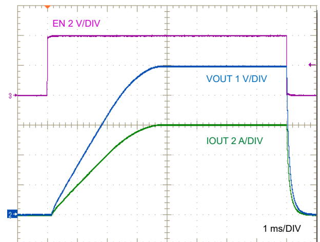
図 8-6. LM644x0-Q1 イネーブルのオン / オフ、6A の抵抗性負荷
