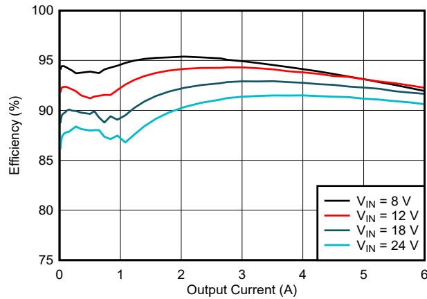
図 8-3. LM644x0-Q1 の効率
