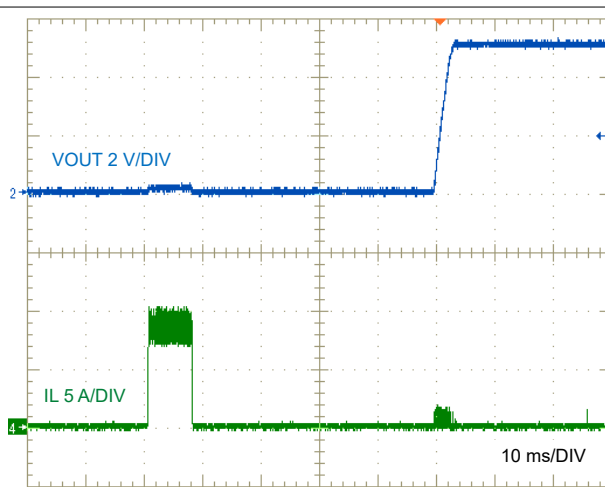
図 7-19. 短絡からの回復
