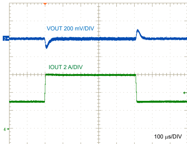
図 8-7. LM644x0-Q1 の負荷過渡、 I_{OUT} = 3A \sim 6A
