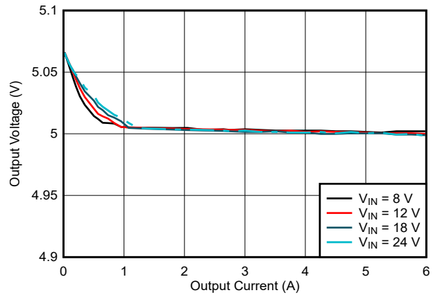
図 8-4. LM644x0-Q1 の負荷およびラインレギュレーション
