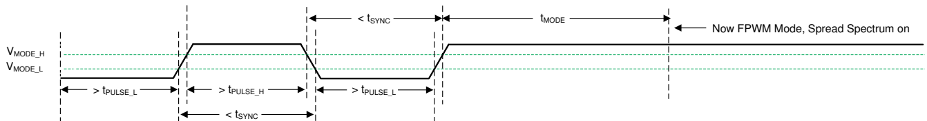
図 7-11. 同期モードから FPWM モードへの遷移
