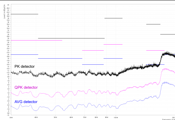
図 8-17. CISPR 25 Class 5 放射 EMI、 バイコニカル アンテナ、水平偏波、 30MHz ~ 200MHz
