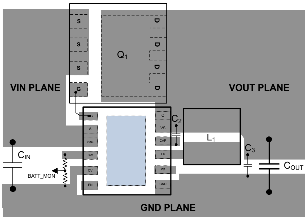
FIG 11-1. LM74721-Q1 Layout Example
