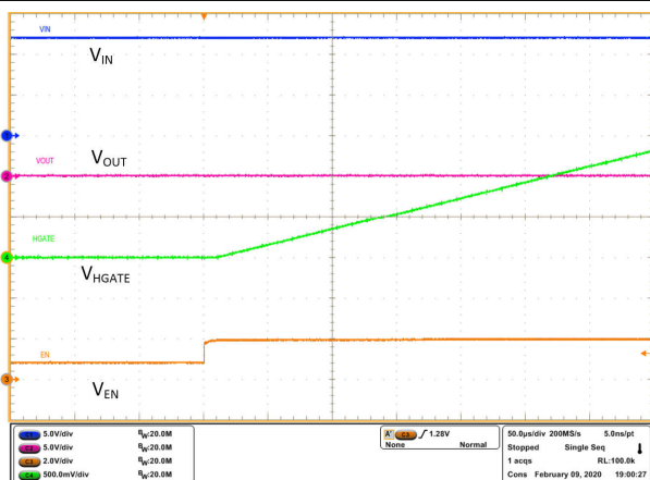
图 9-12. Enable Delay HGATE
