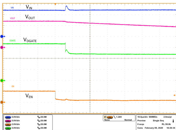
图 9-10. Disable Delay DGATE
