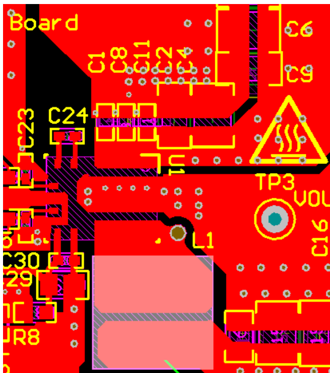
✎ 16. Top Layer
