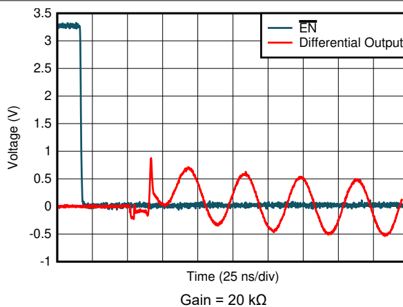
6-24. Turn-On Time
