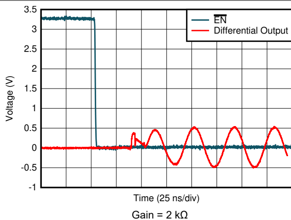
6-23. Turn-On Time
