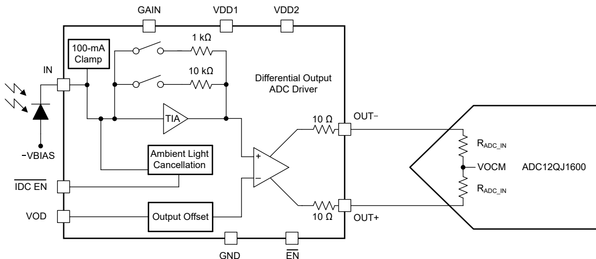
图 8-1. LMH32401-Q1 到 ADC 接口
