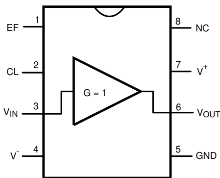
図 3-1. 接続図 : 8 ピン SO PowerPAD
