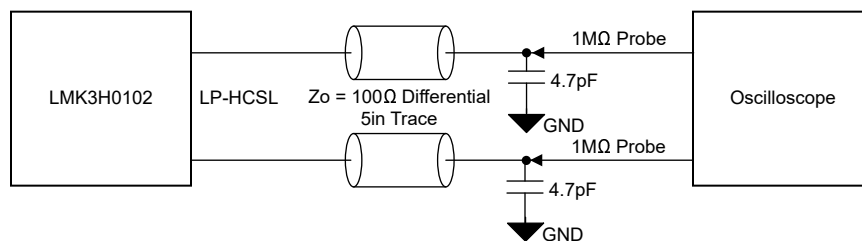
図 6-4. 非 PCIe デバイス テスト時の LP-HCSL 出力の構成
