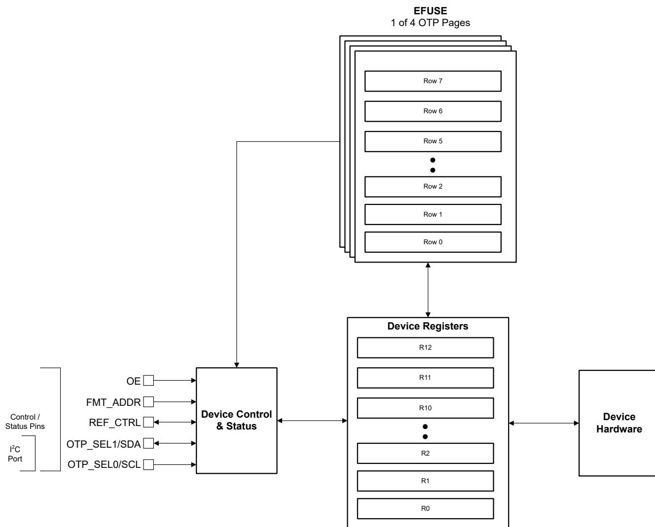
図 7-3. LMK3H0102 のインターフェイスと制御ブロック
