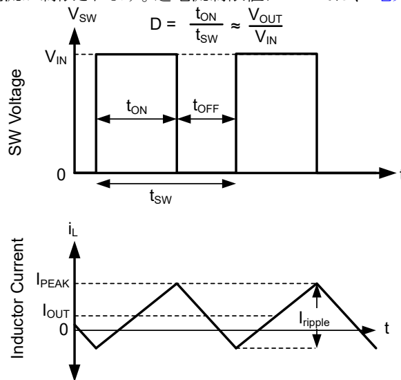
図 7-18. FPWM モード動作
