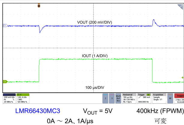
図 8-31. 負荷過渡
