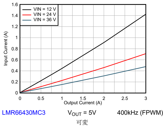
図 8-29. 入力電流と負荷電流との関係
