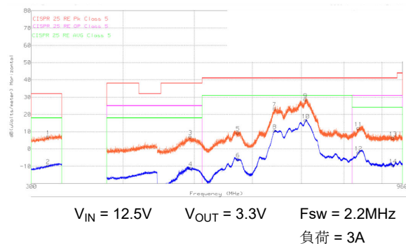
図 8-23. CISPR 25 Class 5 放射 EMI、ログアンテナ、水平偏波、300MHz ~ 960MHz オレンジ：ピーク検出、青：平均検出
