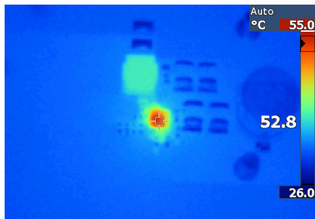
LMQ66430MC3 V_{OUT} = 3.3V 12V_{IN} , 2A, 2.2MHz 固定
