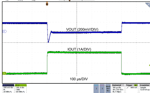
LMQ66430MC3 V_{OUT} = 3.3V 2.2MHz (自動) 0A ~ 2A, 1A/ \mu s 固定
