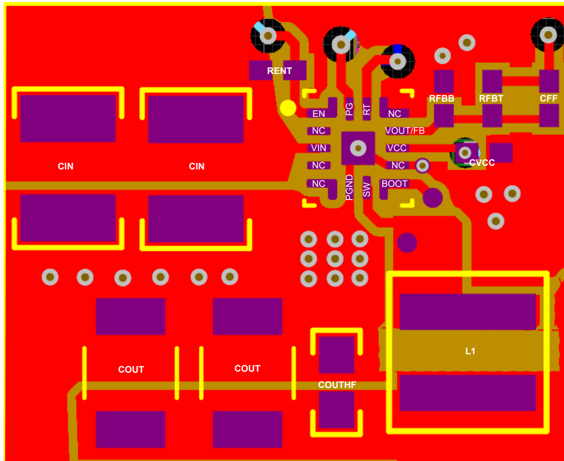
図 8-34. レイアウト例
