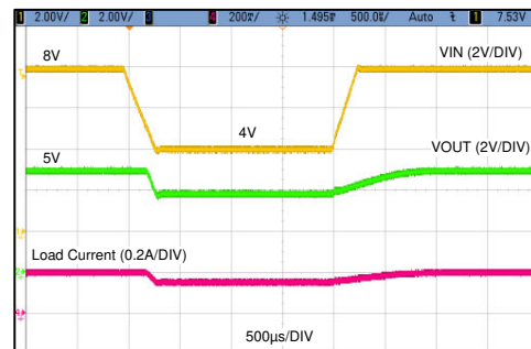
図 7-11. 8V ~ 4V のドロップアウトからの標準的な出力回復
