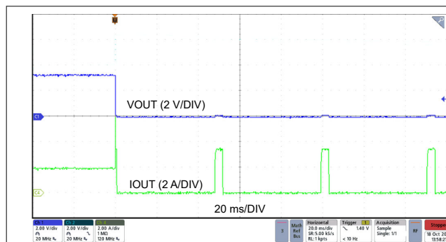
図 7-13. ヒカップの入口
