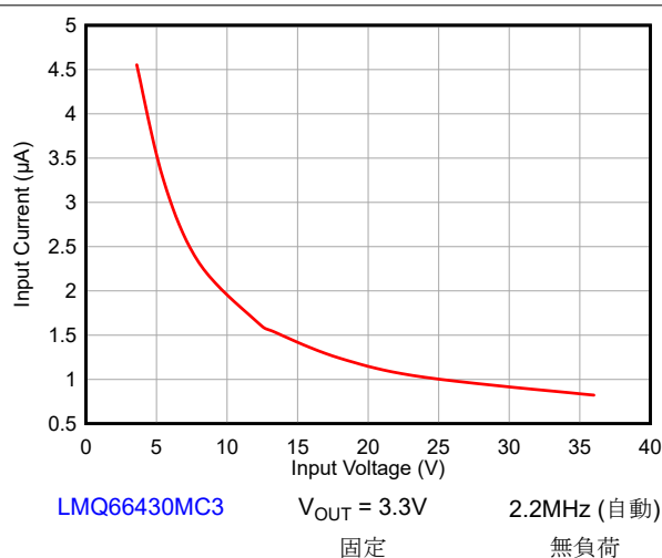
図 8-8. 入力スイッチング電流と入力電圧との関係
