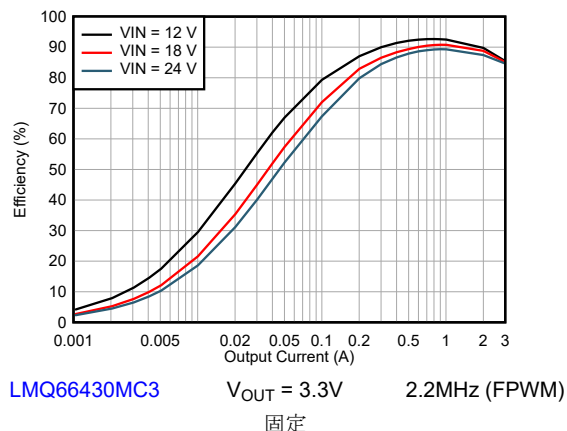
図 8-5. 効率
