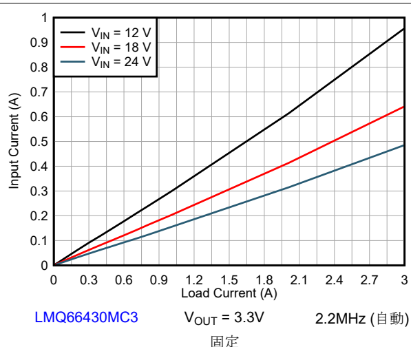
図 8-9. 入力電流と負荷電流との関係
