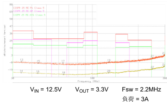
図 8-22. CISPR 25 Class 5 放射 EMI、バイコニカルアンテナ、垂直偏波、30MHz ~ 300MHz オレンジ：ピーク検出、黄：平均検出
