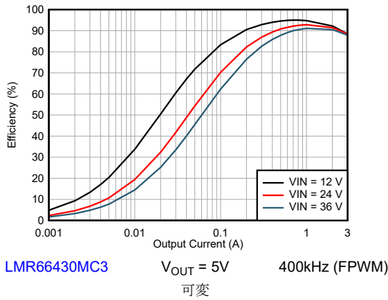
図 8-27. 効率
