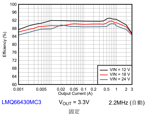
図 8-4. 効率
