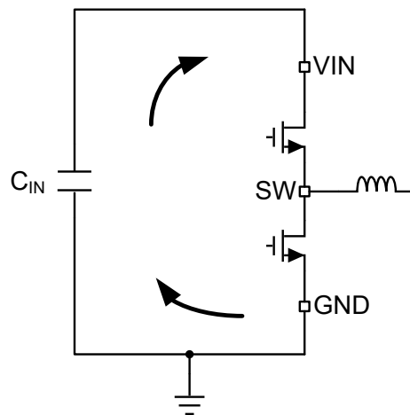
図 8-33. 高速エッジを持つ電流ループ
