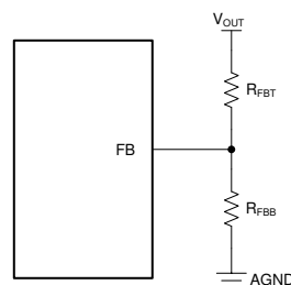
図 7-8. 可変出力バリエーションの出力電圧の設定
