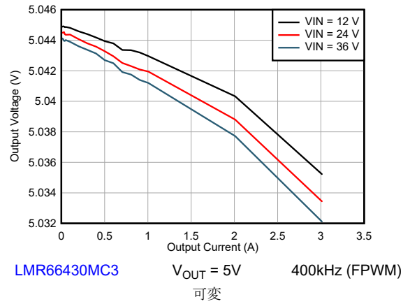
図 8-28. ラインおよび負荷レギュレーション
