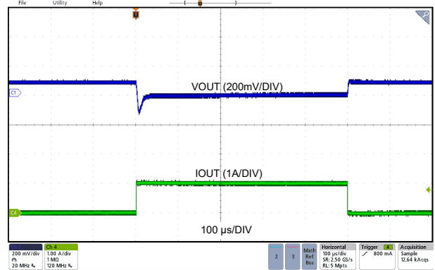
LMQ66430MC3 V_{OUT} = 3.3V 2.2MHz (自動) 0A ~ 1A, 1A/ \mu s 固定
