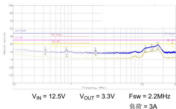
図 8-20. CISPR 25 Class 5 放射 EMI ロッドアンテナ、 150kHz ~ 30MHz 青：ピーク検出、黄：平均検出
