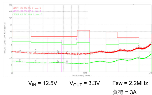
図 8-21. CISPR 25 Class 5 放射 EMI、バイコンカルア ンテナ、水平偏波、30MHz ~ 300MHz 赤：ピーク検出、緑：平均検出
