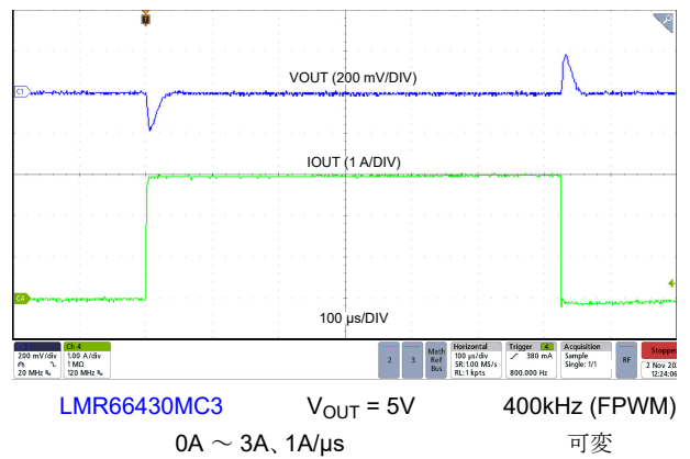
図 8-30. 負荷過渡
