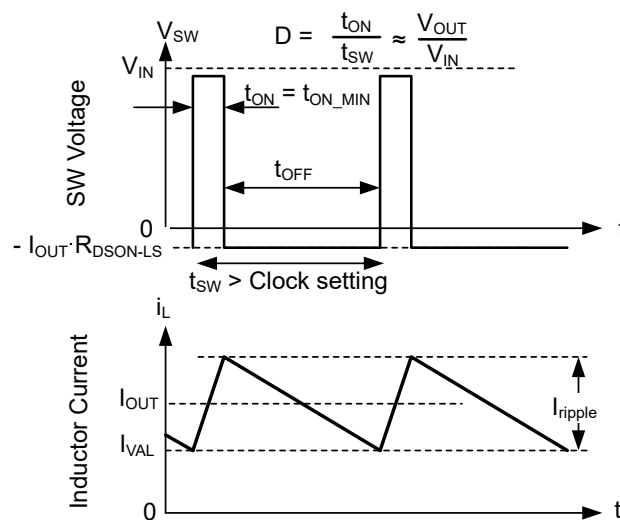
図 7-19. バレー電流モード動作
