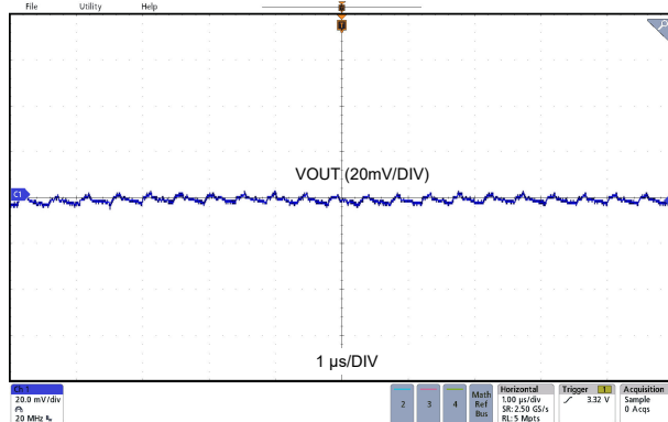
LMQ66430MC3 V_{OUT} = 3.3V 2A 負荷 固定
