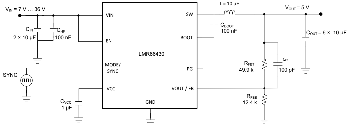
図 8-26. アプリケーション回路 2 - 5V (可変)、3A、400kHz
