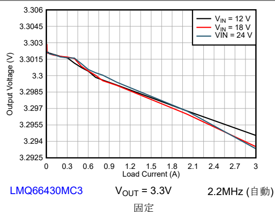
図 8-7. ラインおよび負荷レギュレーション
