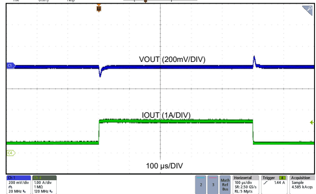
LMQ66430MC3 V_{OUT} = 3.3V 2.2MHz (自動) 0.5A ~ 1.5A, 1A/ \mu s 固定
