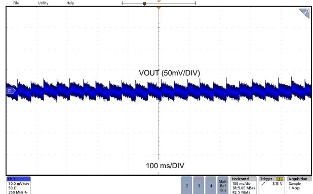
LMQ66430MC3 V_{OUT} = 3.3V 無負荷 固定
