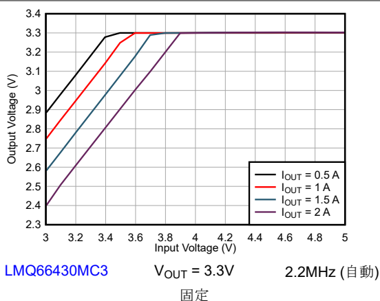
図 8-6. ドロップアウト
