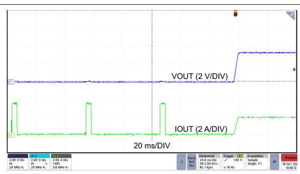
図 7-14. ヒカップの出口
