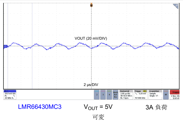
図 8-32. 出力電圧リップル
