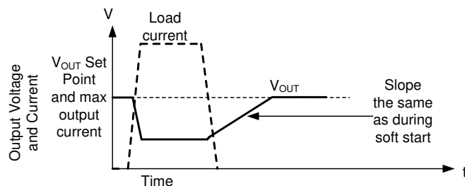
図 7-10. ドロップアウトからの回復
