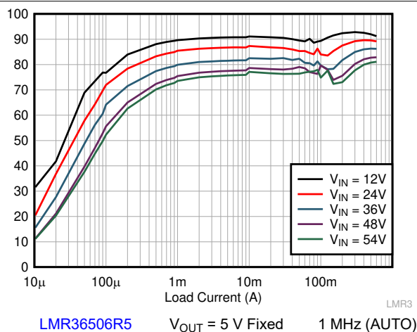
图 9-8. Efficiency
