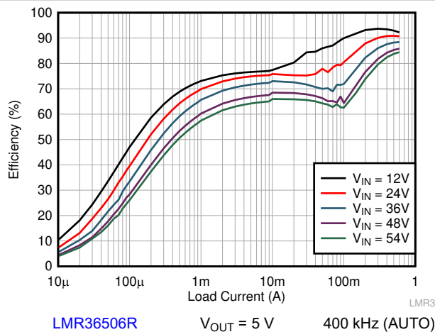
图 9-6. Efficiency
