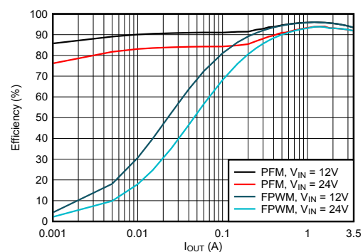
効率と出力電流との関係 V_{\text{OUT}} = 5\text{V} 、 440\text{kHz}
