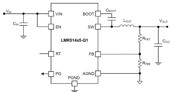
概略回路図
