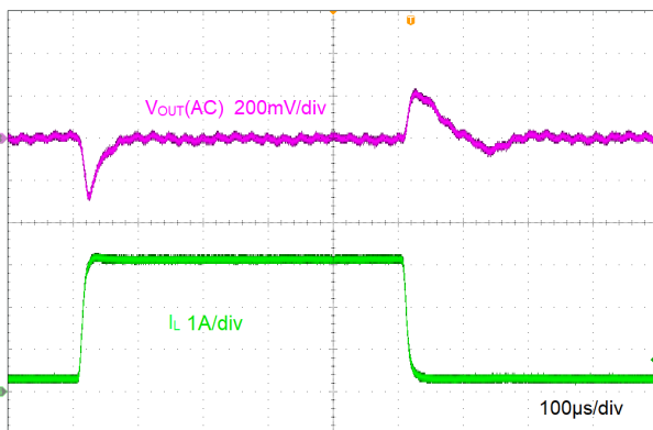
8-6. Load Transient
