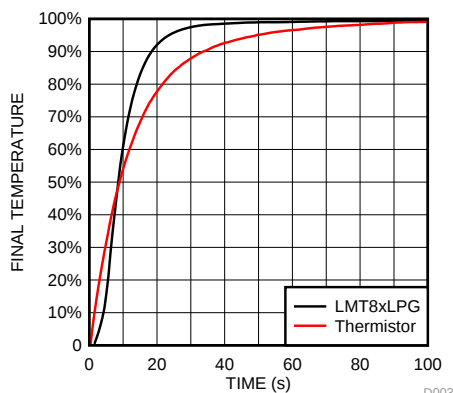
熱時定数
