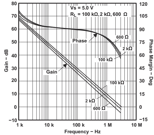
図 6-2. LMV321 の周波数応答と抵抗性負荷との関係
