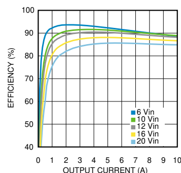
25°Cにおける 3.3V 出力の効率
