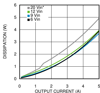
図 5-36. 85°Cの周囲温度における 0.8V 出力の消費電力
