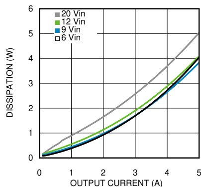
図 5-32. 85°Cの周囲温度における 1.2V 出力の消費電力
