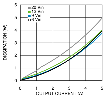
図 5-34. 85°Cの周囲温度における 1V 出力の消費電力
