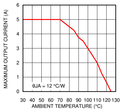
図 5-38. 温度ディレーティング
