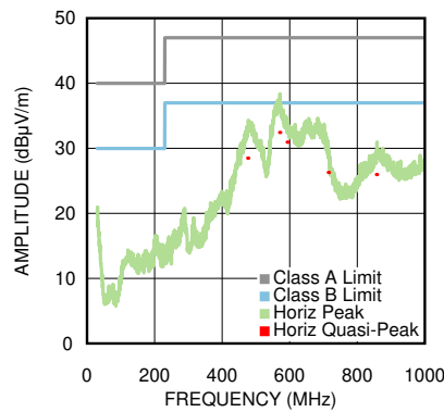
図 7-6. デモ ボードの放射 EMI (EN 55022) (AN-2125 を参照)
