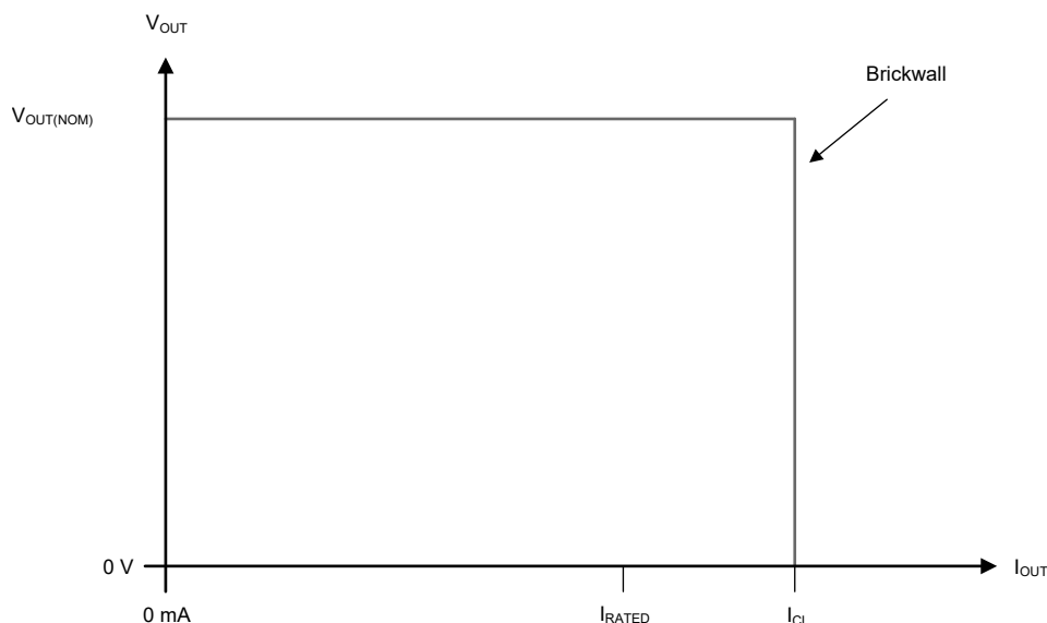
図 6-3. Current Limit
