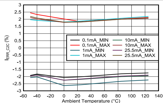
図 6-4. チャネル間の電流精度と温度との関係 (MC = 0)
