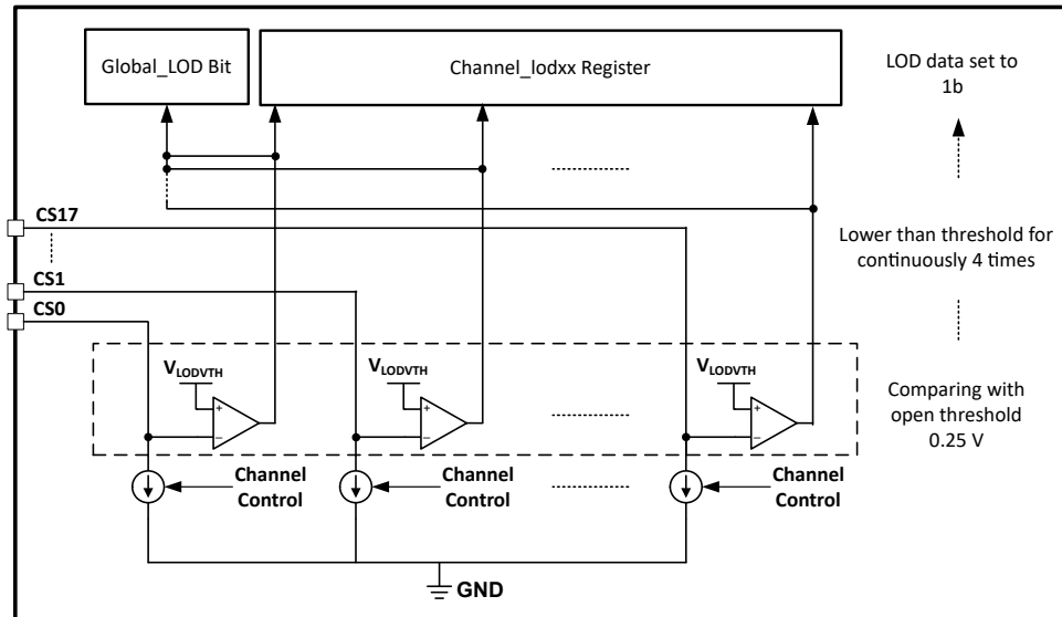
8-11. LOD Circuits
