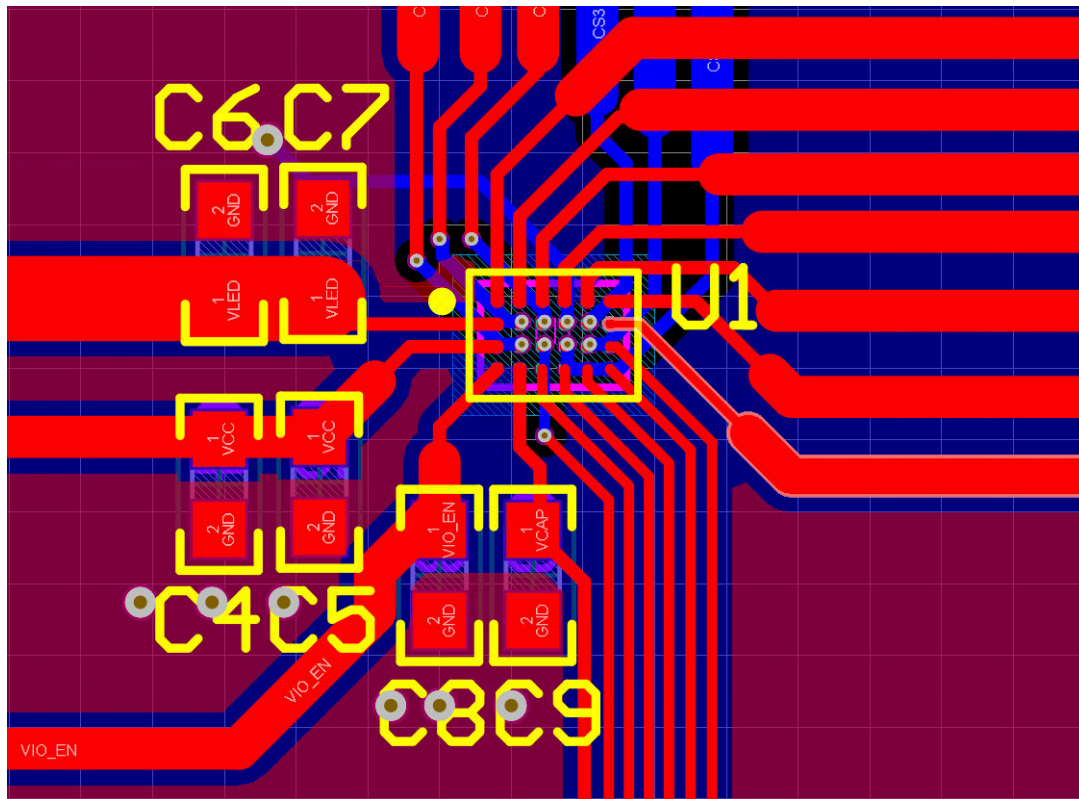
図 9-10. LP5867 Layout Example
