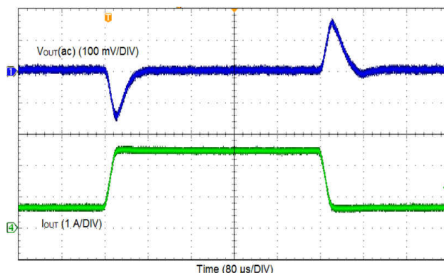
图 9-5. DCM Mode
