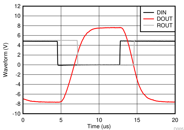
図 7-2. Loopback Waveforms
