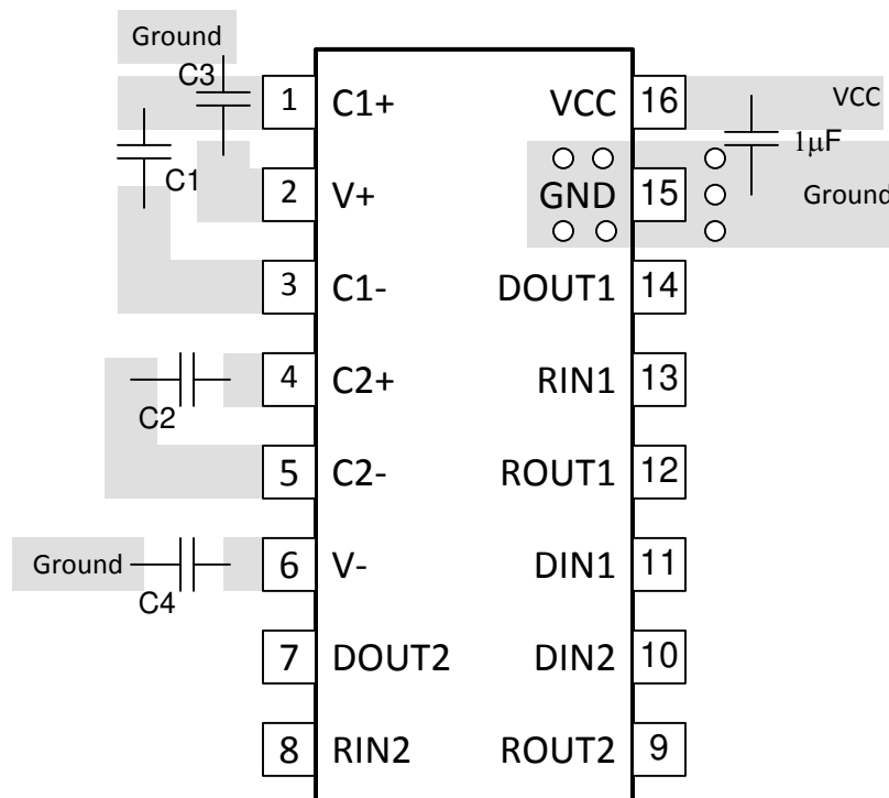
図 7-3. MAX232E Layout
